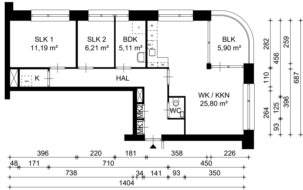
Plattegrond type D
