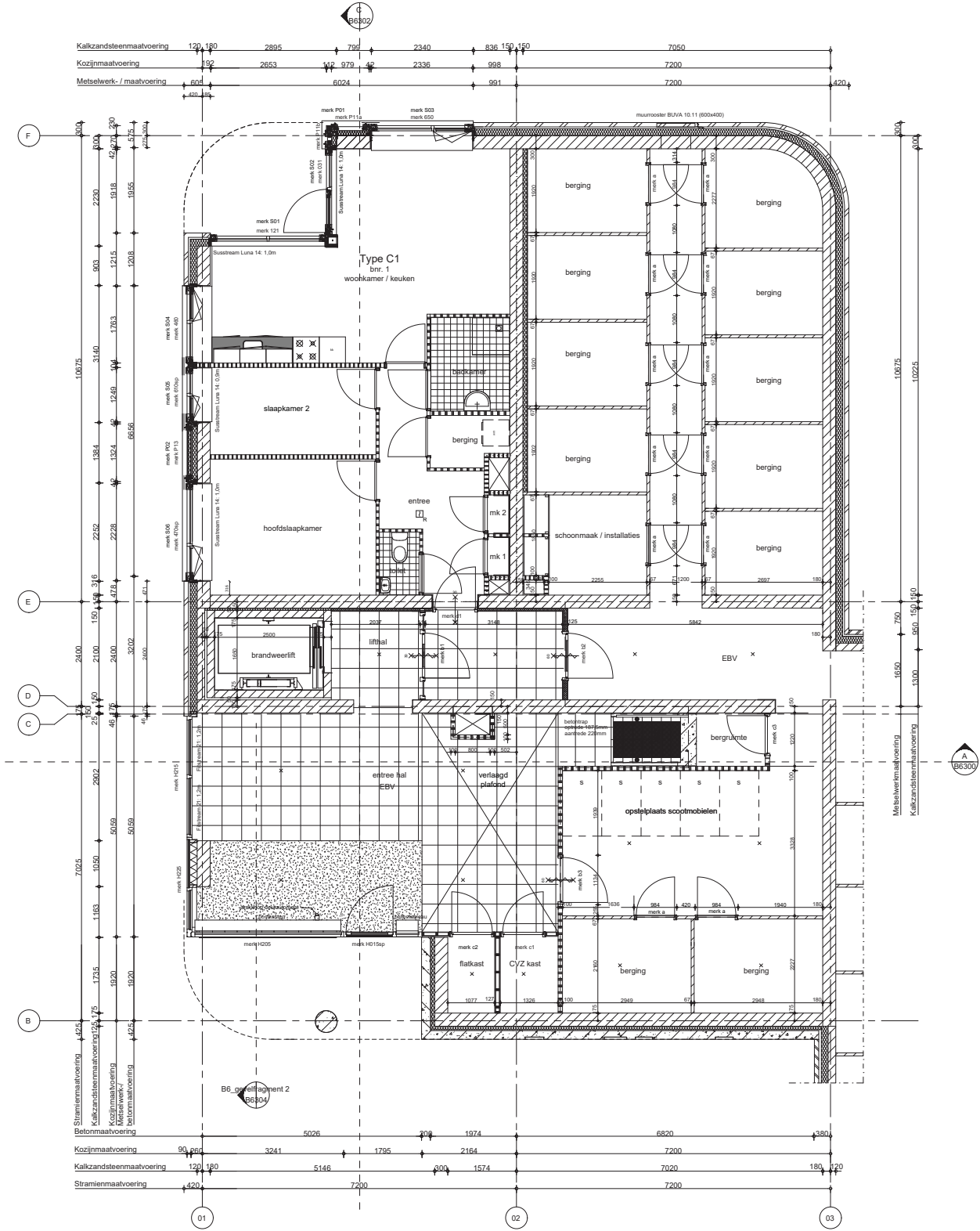
Plattegrond berging laagbouw
